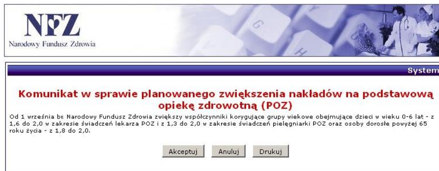
Rys. 2.3 Komunikat świadczeniodawcy
